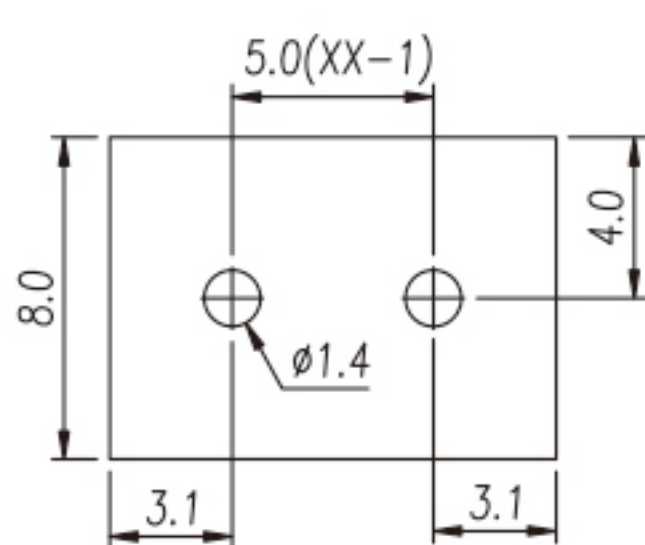
P.C.B. LAYOUT
