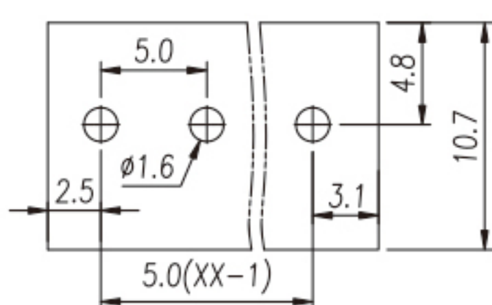
P.C.B. LAYOUT
