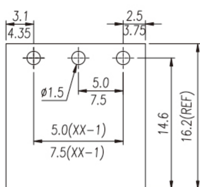
P.C.B. LAYOUT
