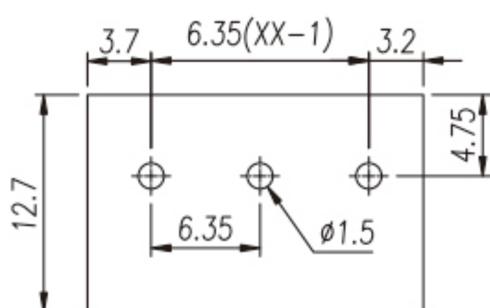
P.C.B. LAYOUT
