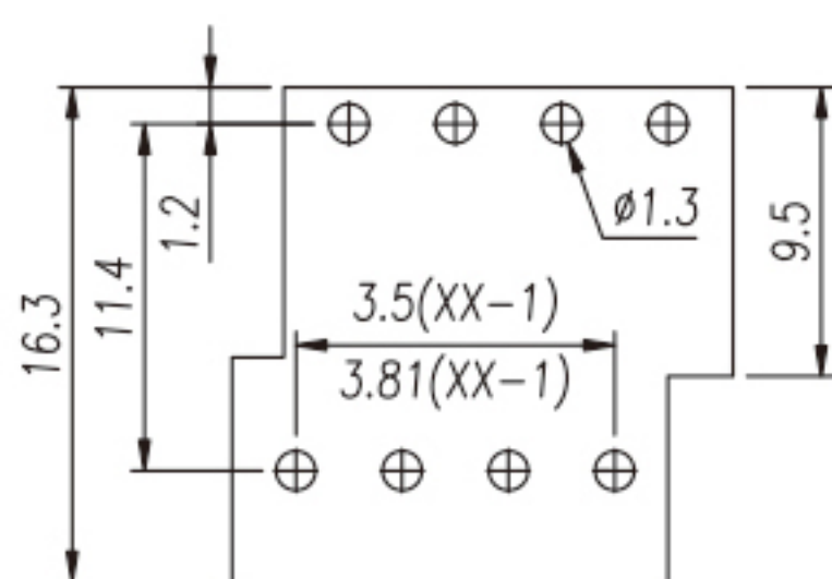
P.C.B. LAYOUT
