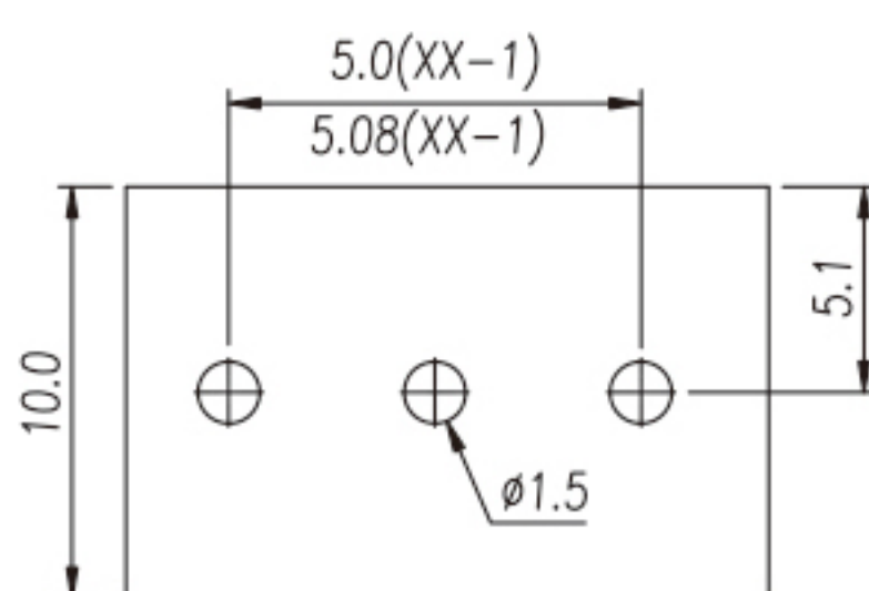
P.C.B. LAYOUT
