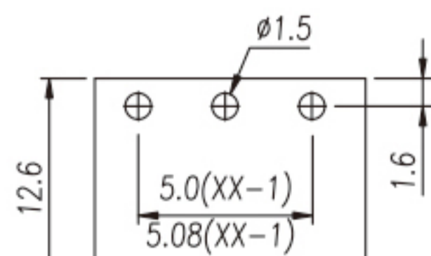
P.C.B. LAYOUT
