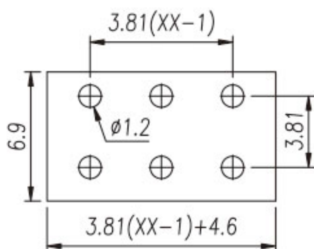
P.C.B. LAYOUT
