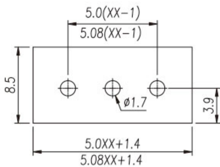
P.C.B. LAYOUT
