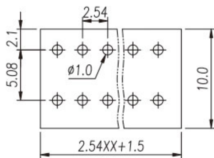
P.C.B. LAYOUT
