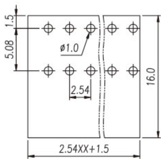
P.C.B. LAYOUT
