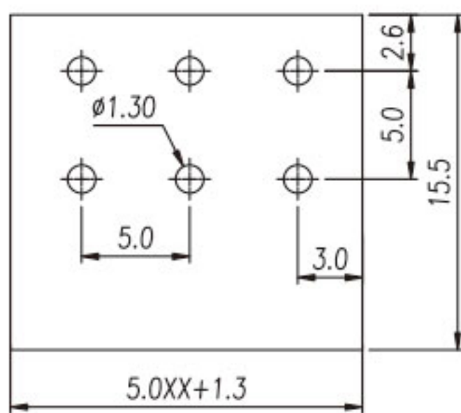
P.C.B. LAYOUT
